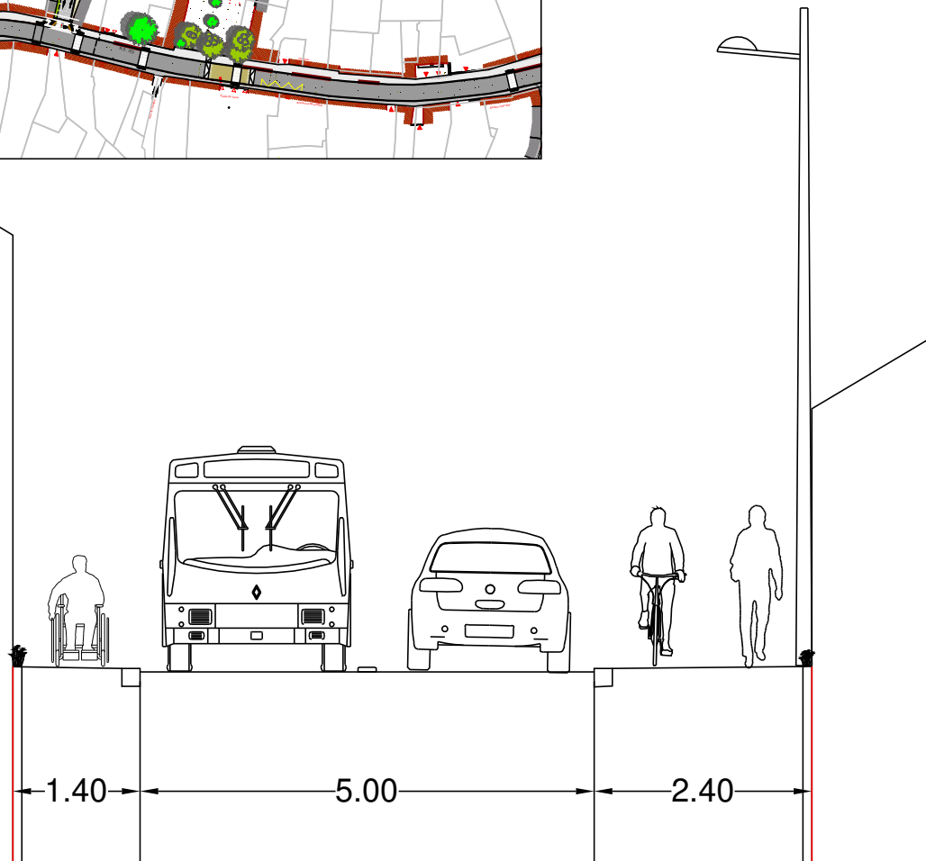
Profil route de Paimboeuf - 'La Ville' mini Scénario, voie verte urbaine
