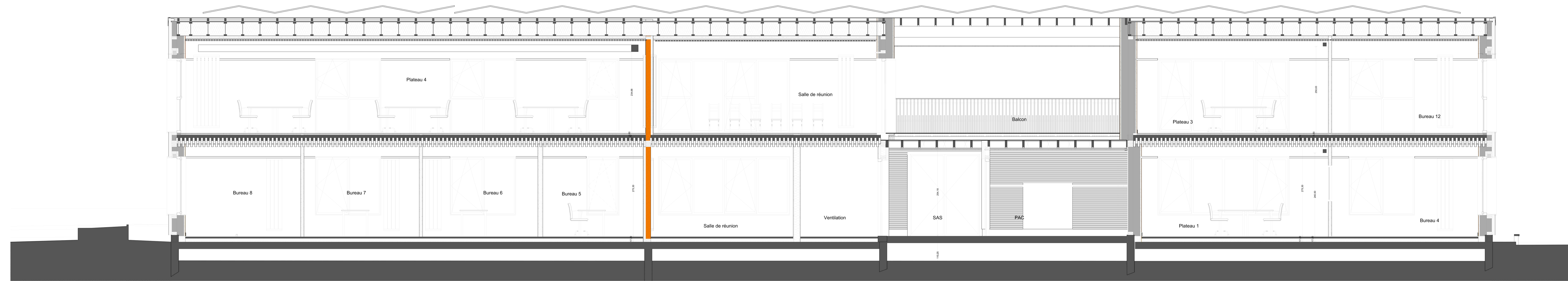
Coupe 5 1:50
