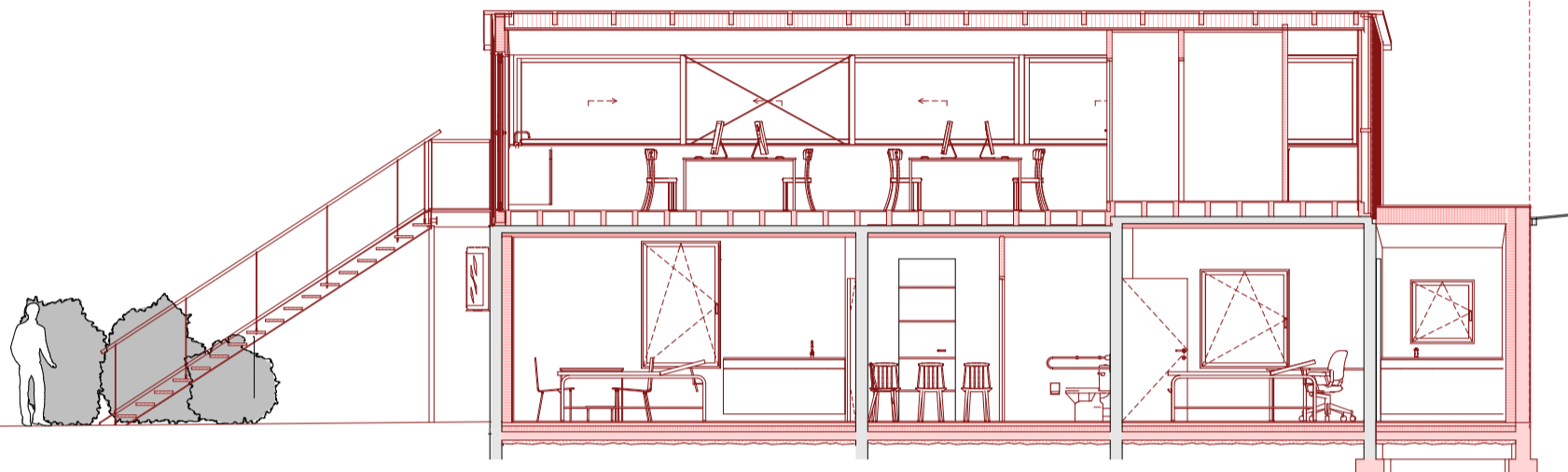
Coupe longitudinale Echelle 1-100e
