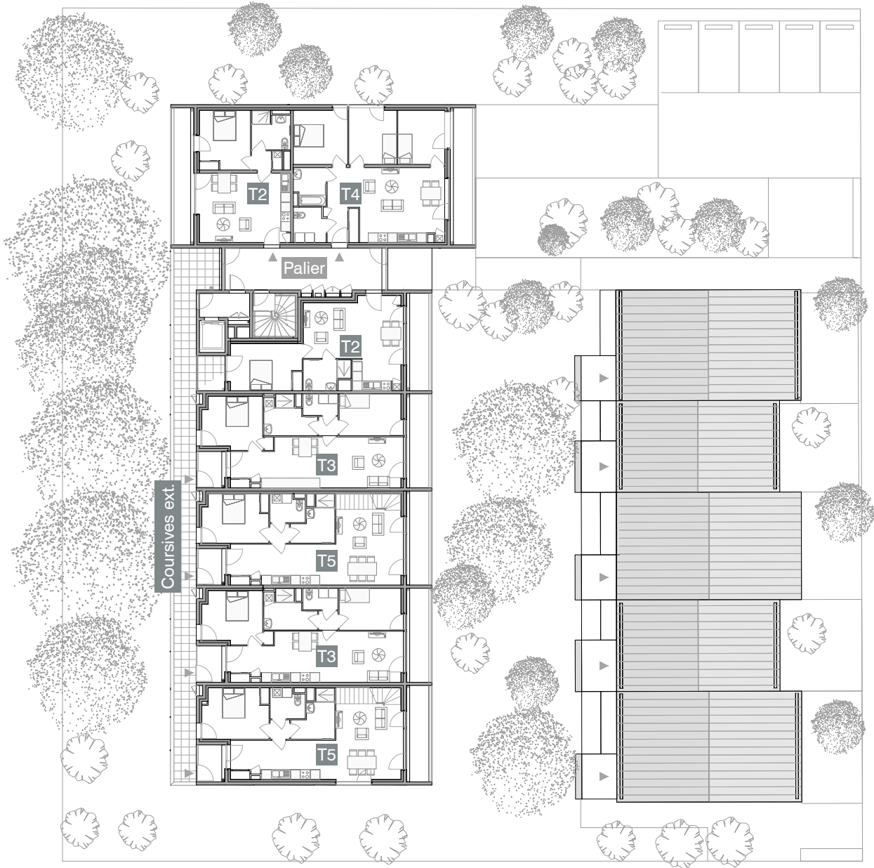
PLAN NIVEAU 2
