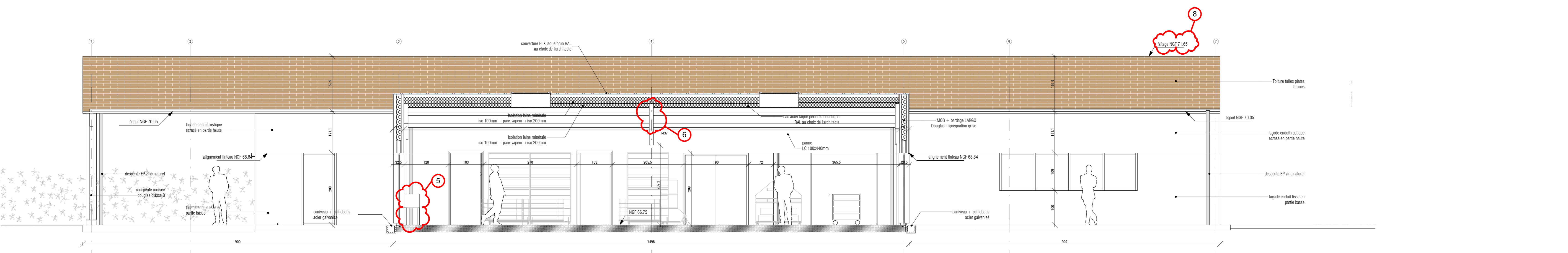
Coupe CC Ech : 1 : 50
