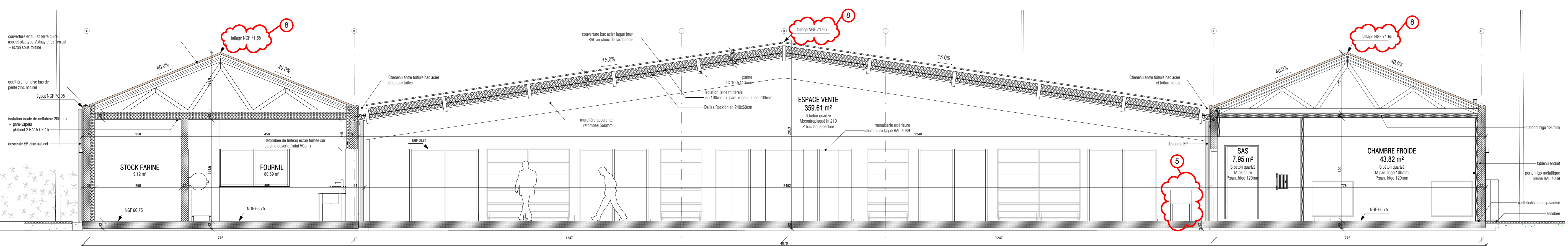
Coupe BB Ech : 1 : 50
