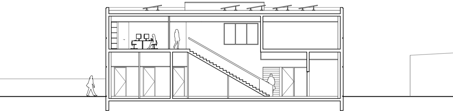
Coupe BB
