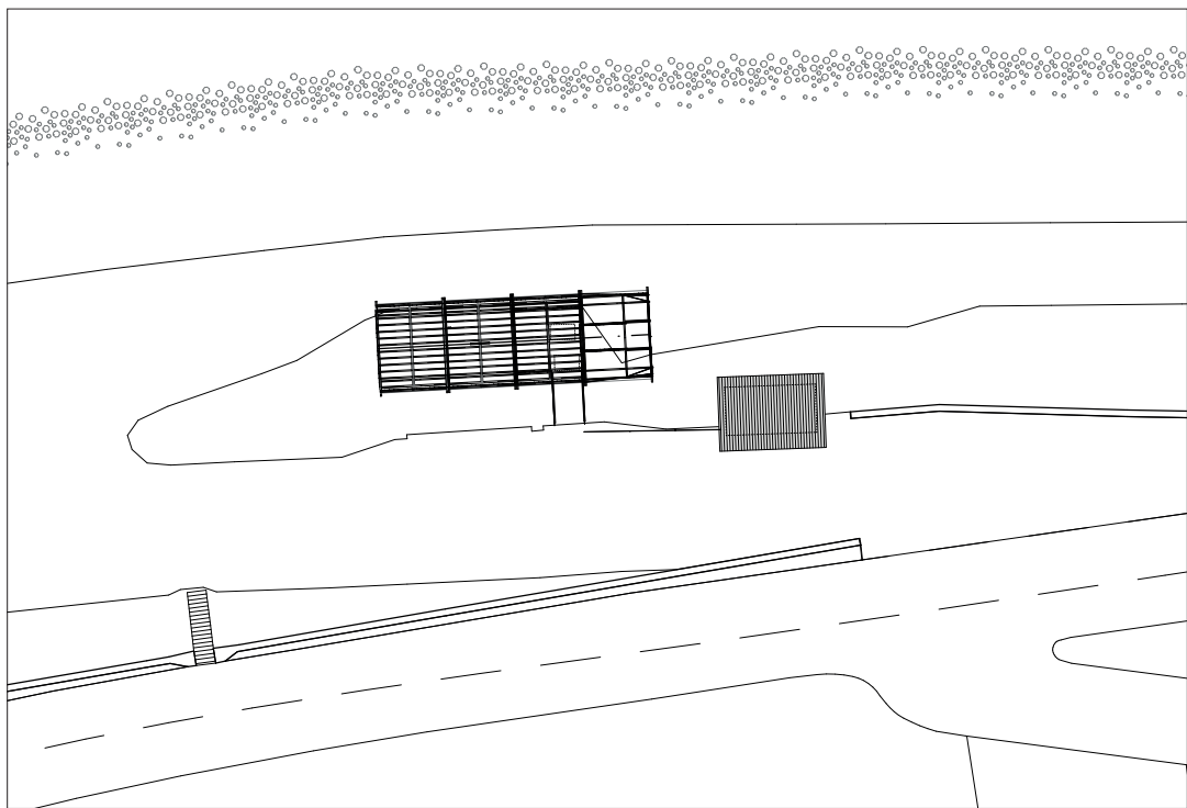
Plan masse _ 1/500 ☉ 10
