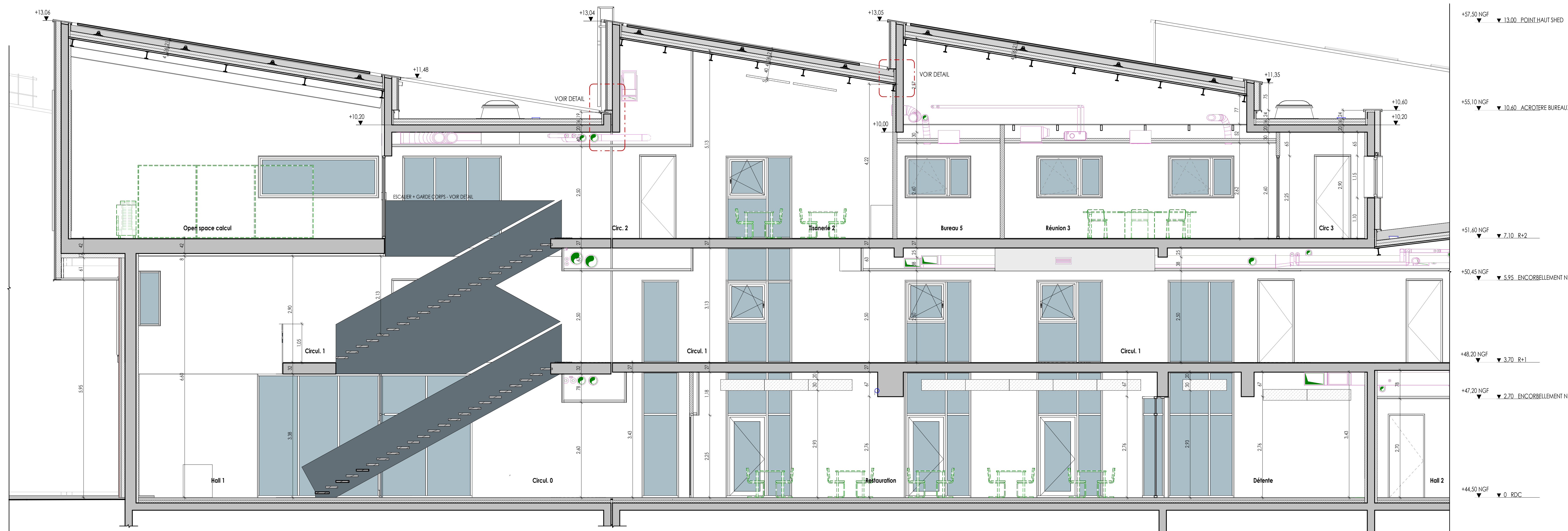
COUPE B Echelle : 1 : 50
