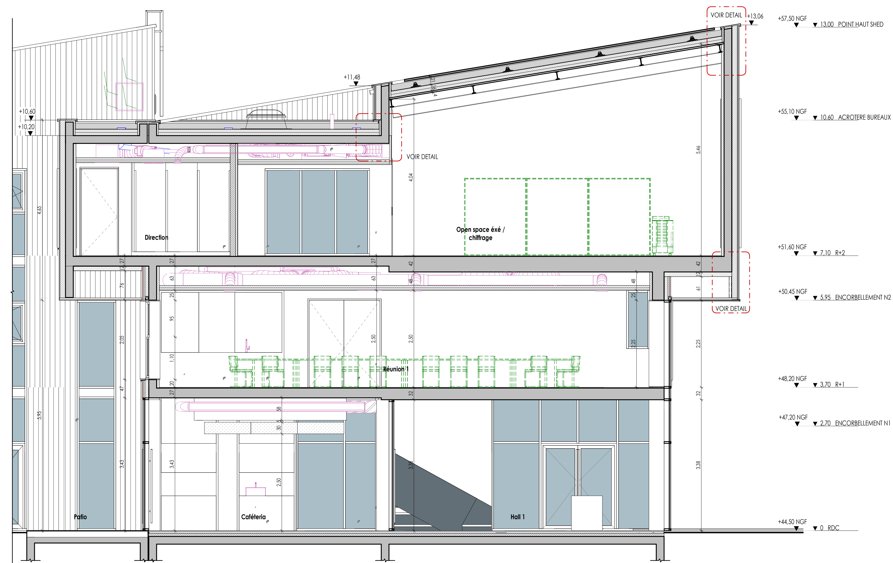
COUPE A1 Echelle : 1 : 50
