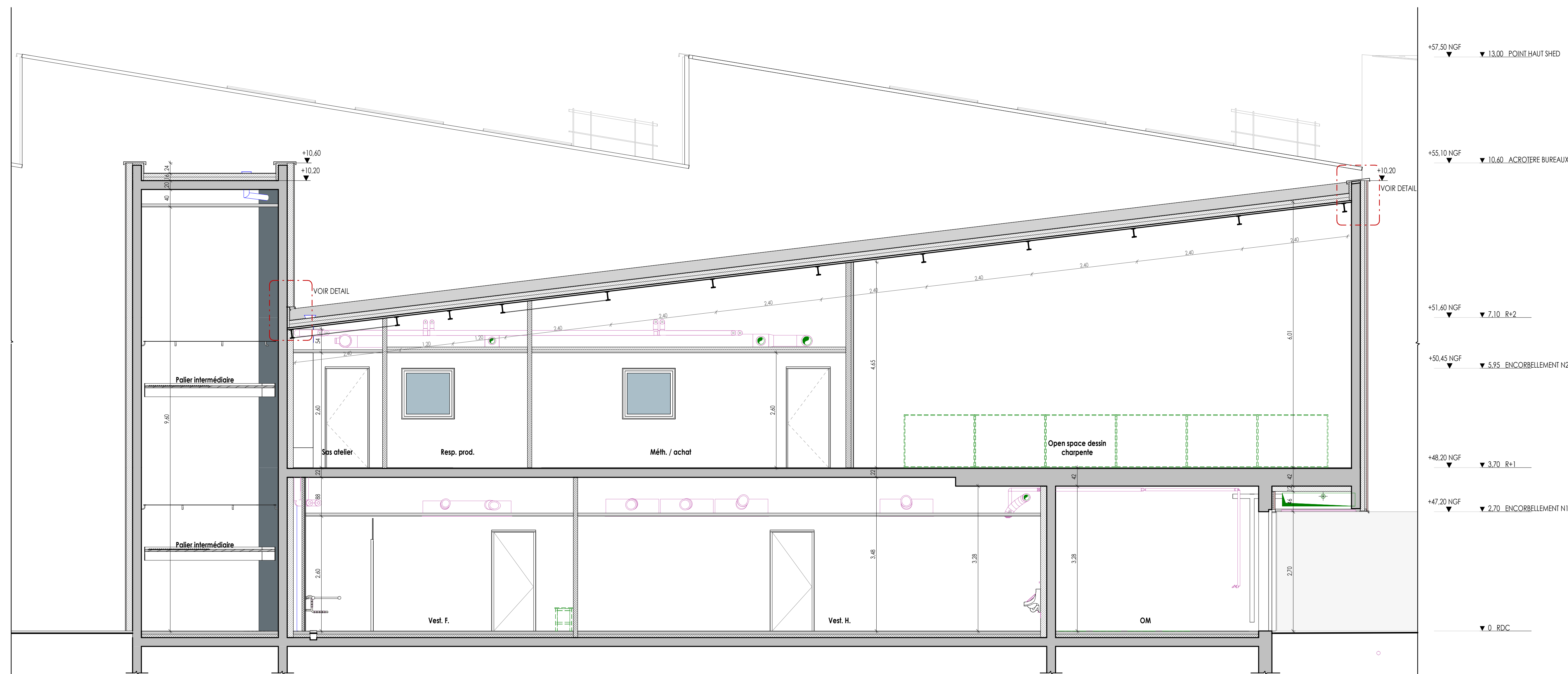
COUPE A2 Echelle : 1 : 50
