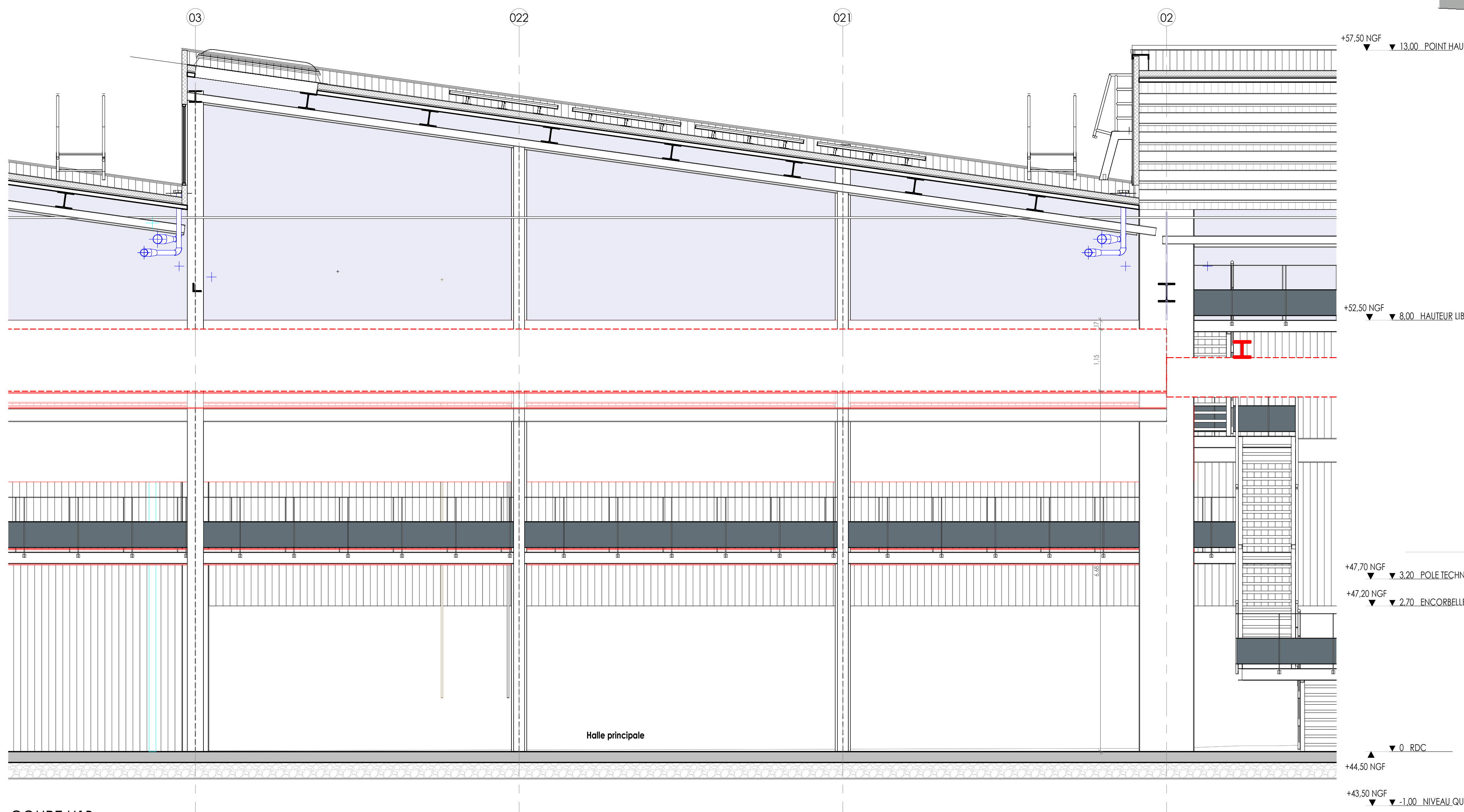
COUPE U1B Echelle : 1 : 50
