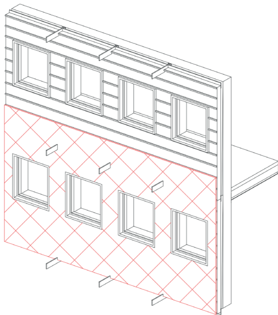
4. bardage
